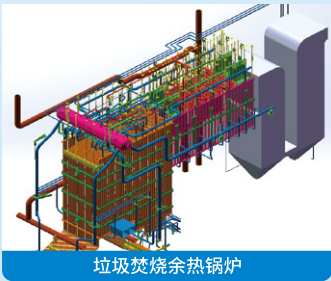
垃圾焚烧余热锅炉
