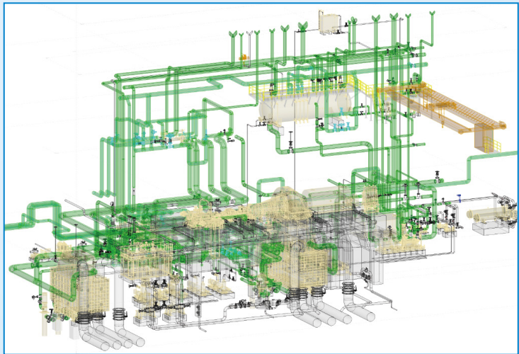
深圳光明余热发电—超高压一次再热汽轮发电机组
